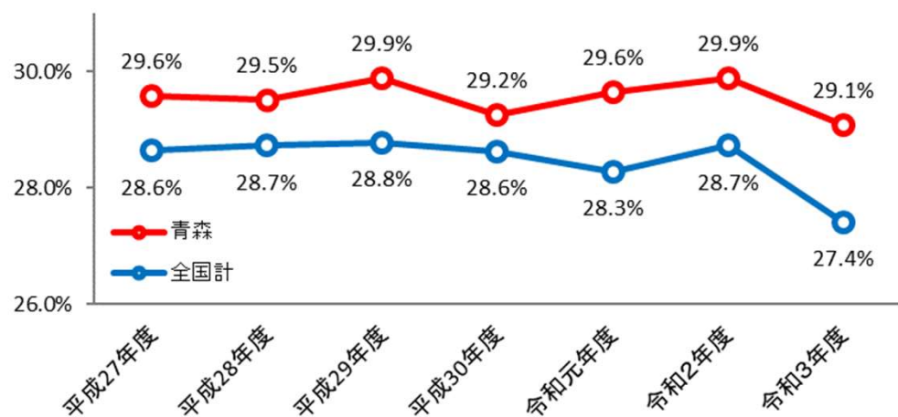
中性脂肪 \geq 150mg/dlの者の割合等(男性)
